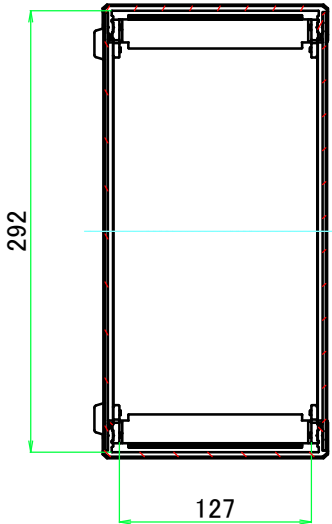
A-A (1:5)
